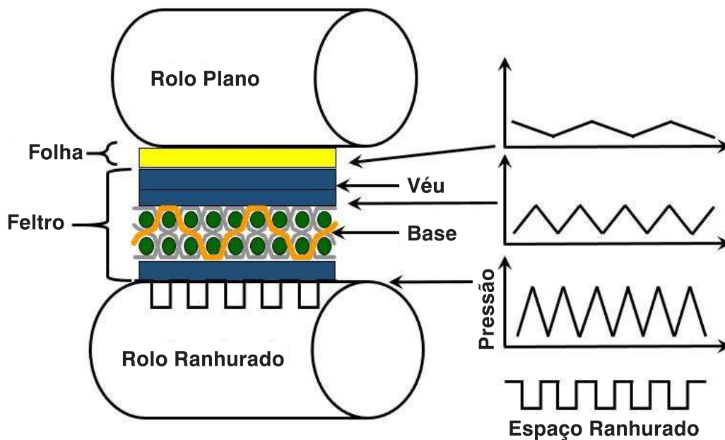
Figura 9: Nipa da prensa.
