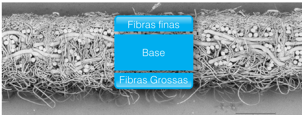
Figura 1: Corte transversal de um feltro úmido.
