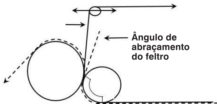
Figura 5: Geometria de prensa.
