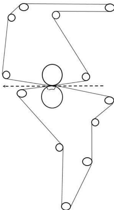
Figura 7: Geometria de dupla feltragem.
